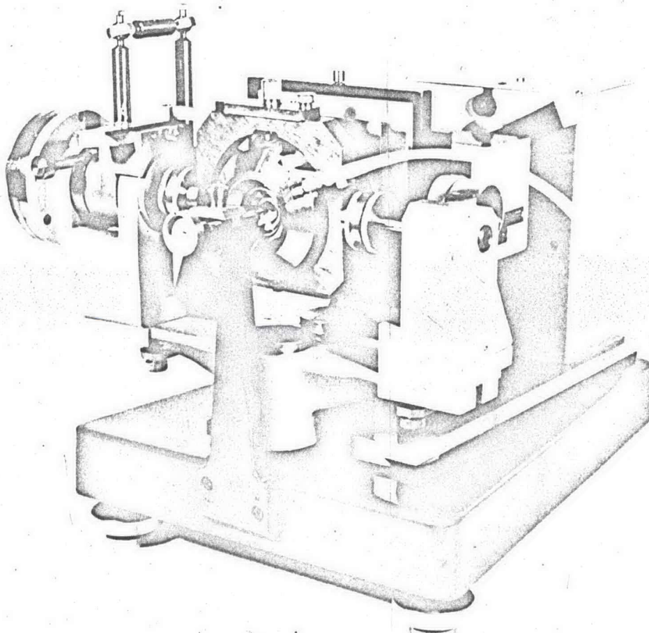
Fig. 2 - Chambre à précession pour les études de diffraction X sous pression
